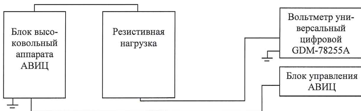
Рисунок 2 - Схема определения относительной основной погрешности измерений силы переменного тока промышленной частоты
